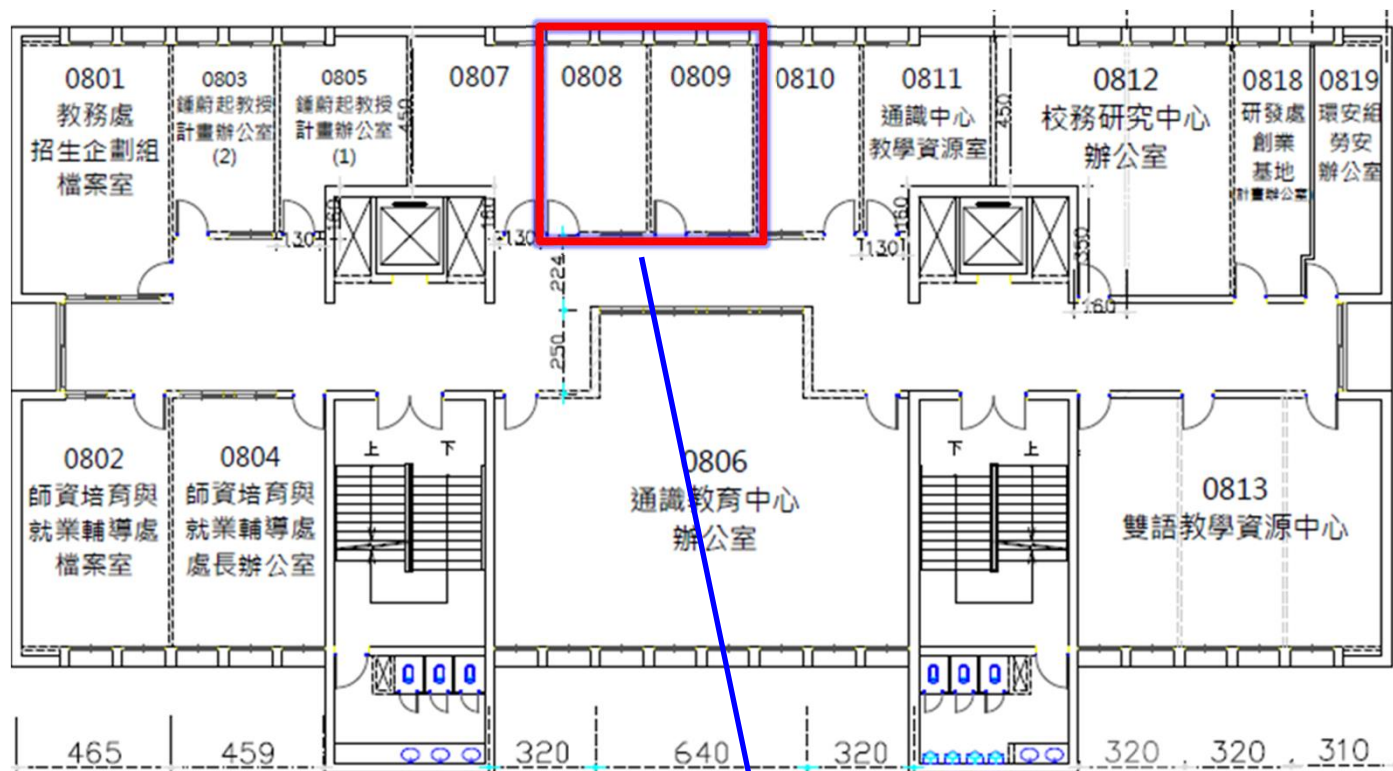
行政大樓 八樓平面圖 (單位:公分)
