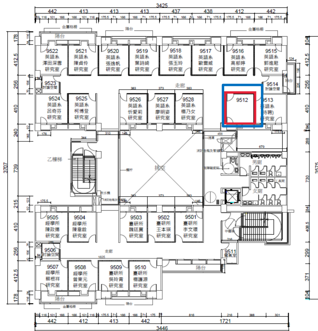
新研究大樓 伍層平面圖 (單位:公分)
