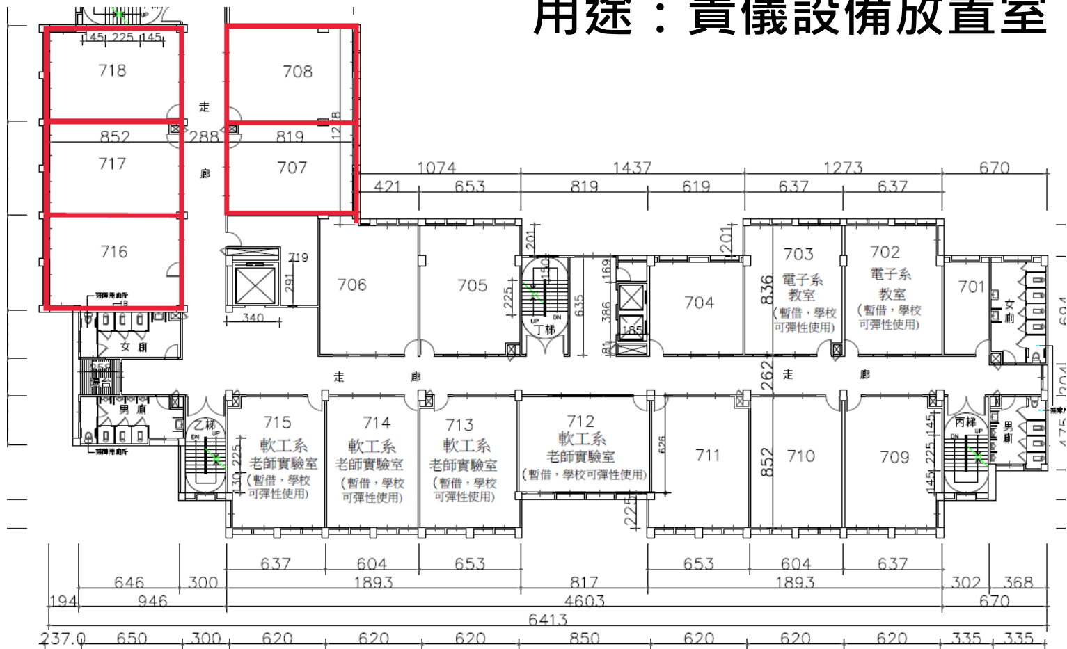
高斯大樓 七樓平面圖 (單位：公分)
