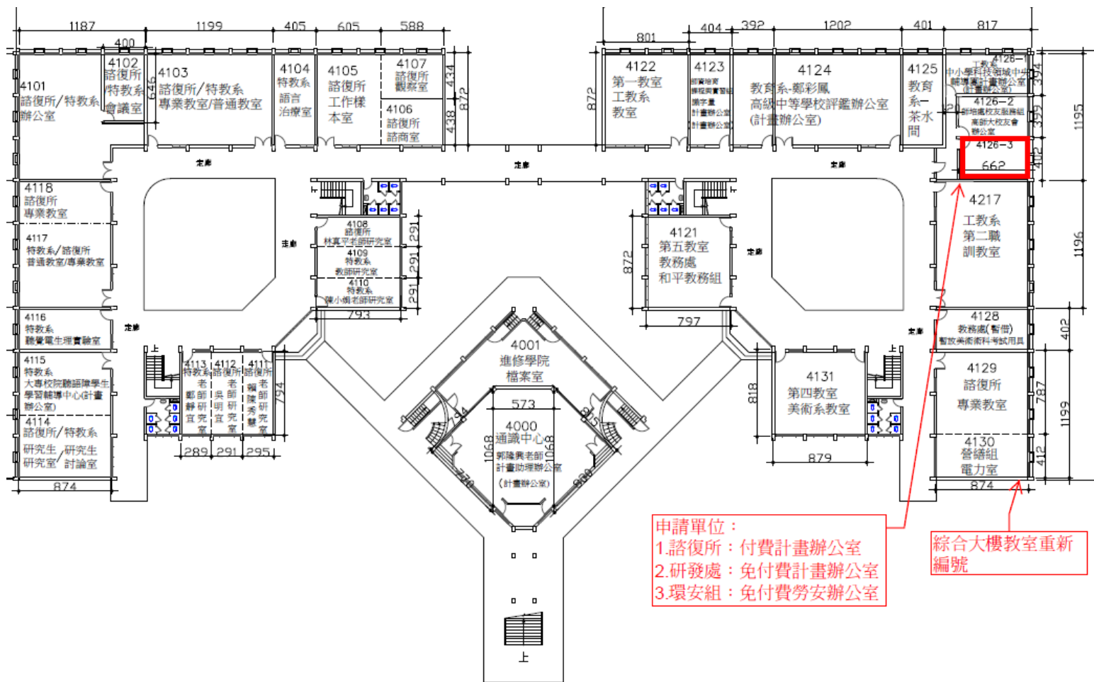
綜合大樓一樓平面圖 單位: 公分
