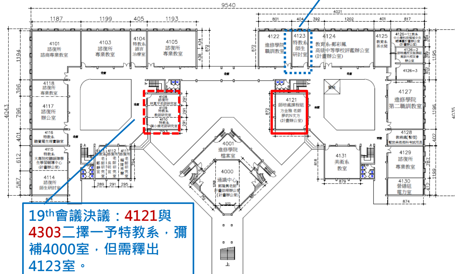
綜合大樓一樓平面圖 單位：公分
