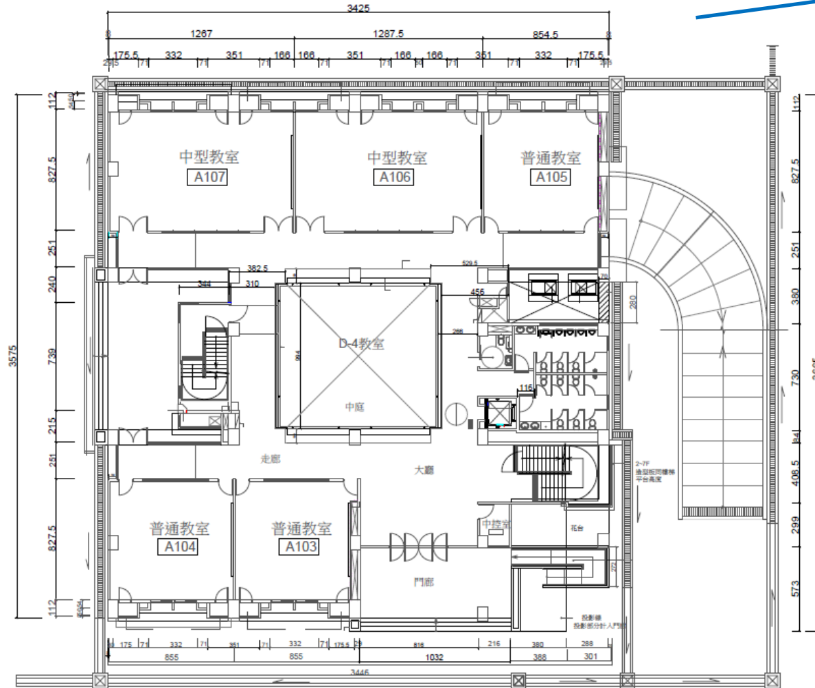
壹層平面圖(單位:公分)
