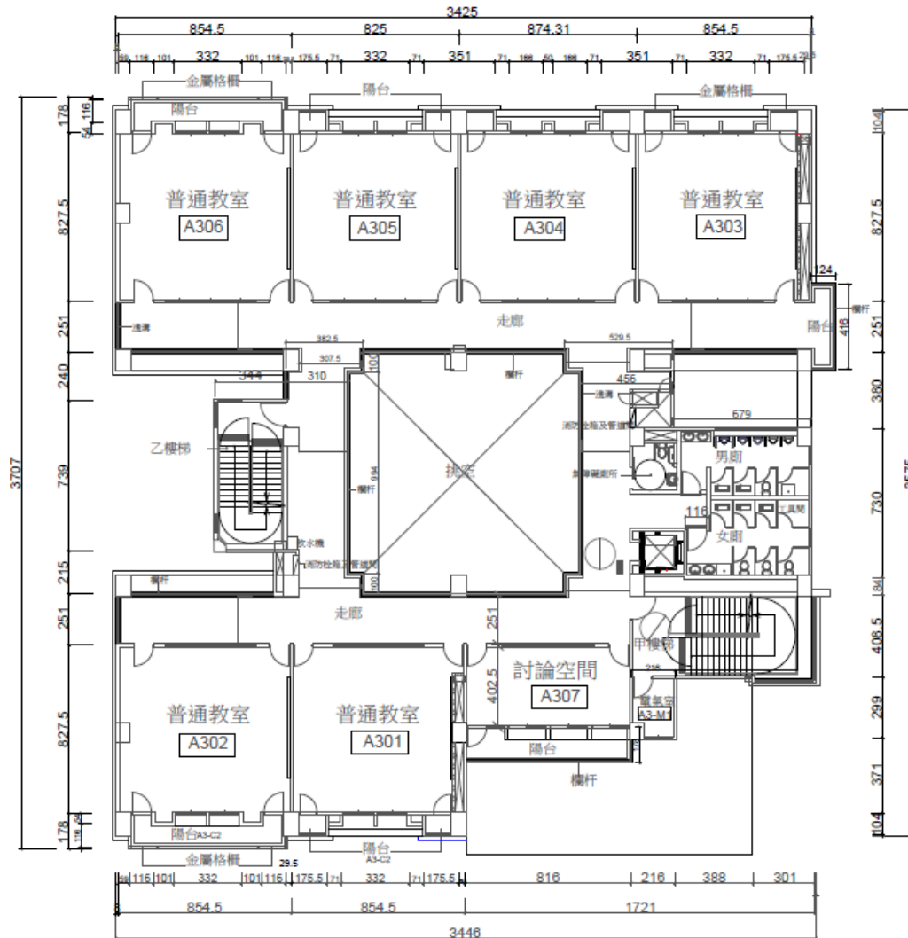
參層平面圖(單位:公分)
