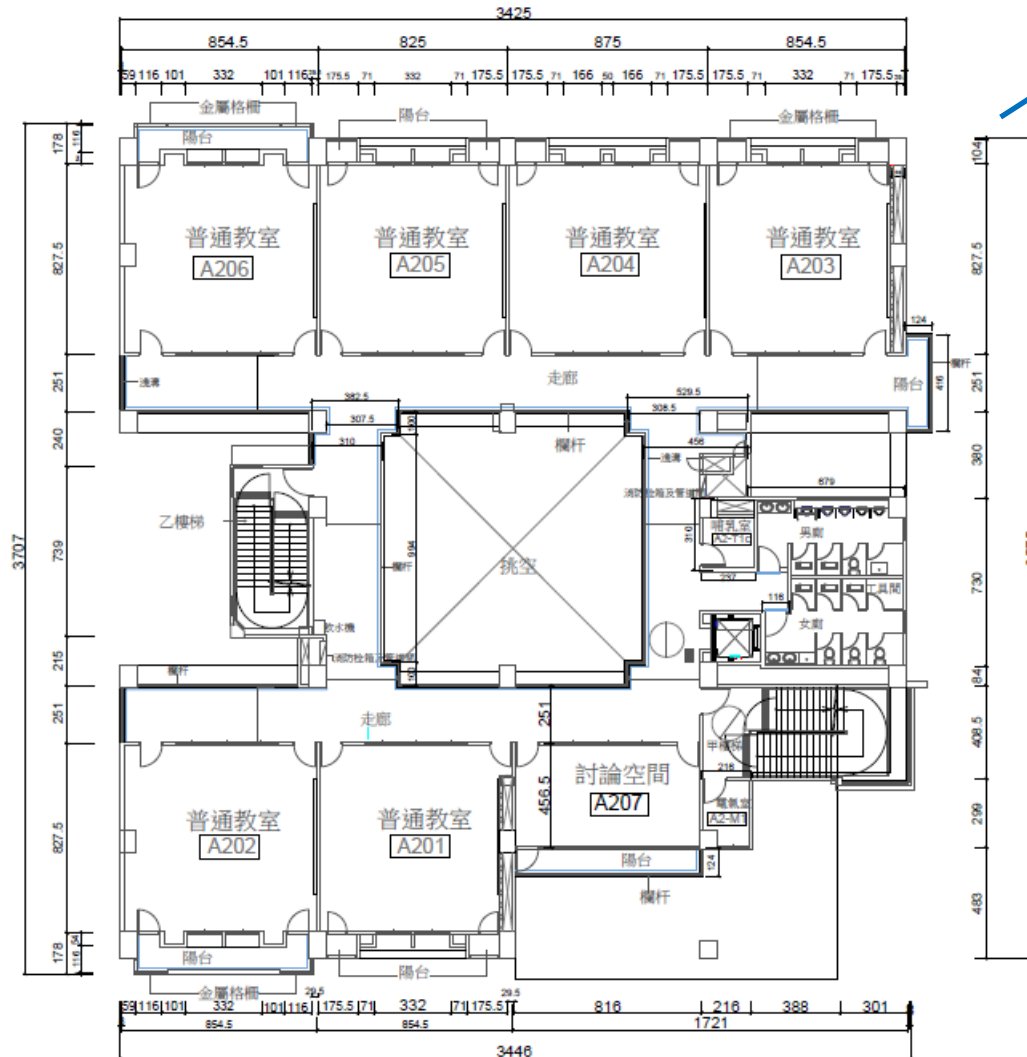
貳層平面圖 (單位:公分)
