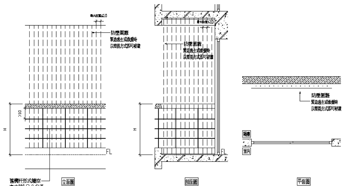
圖例十七 陽臺欄杆架設防壁圍籬
