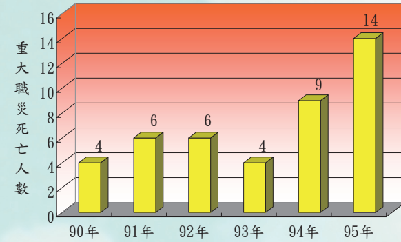
營造業泥作作業重大職業災害統計圖
