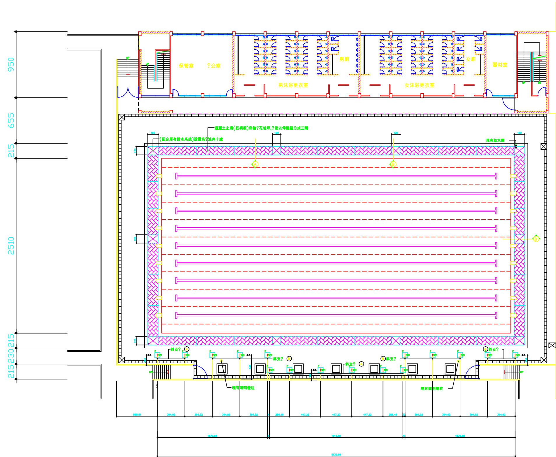
壹層平面圖 S=1:150
