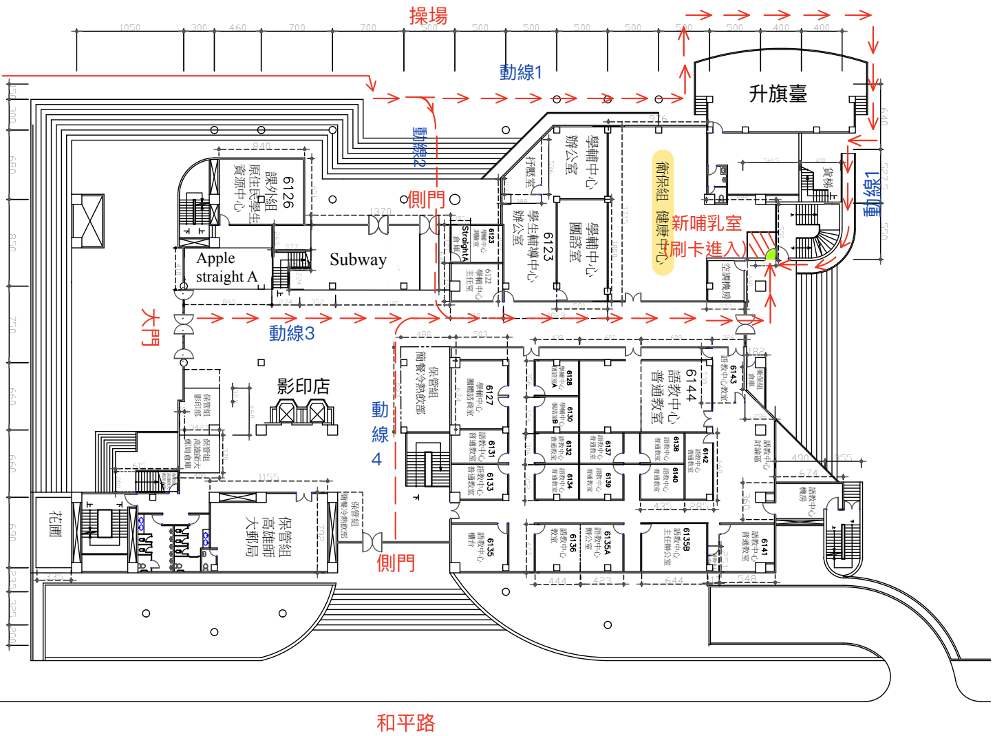
活動中心一樓平面圖 單位：公分
